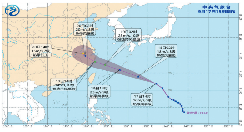
今年第14号台风“普拉桑”未来72小时路径概率预报图 2024年9月17日14时-20日14时(北京时间)
