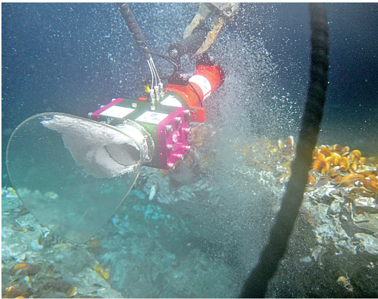
采火装置在海底冷泉喷口采集可燃冰(9月18日摄)。(广州海洋地质调查局供图)
